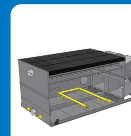
Wateragitatiesysteem
