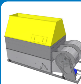
Uitblaasplenum
