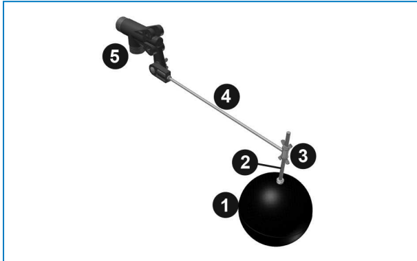
Frishwasserventilbaugruppe
